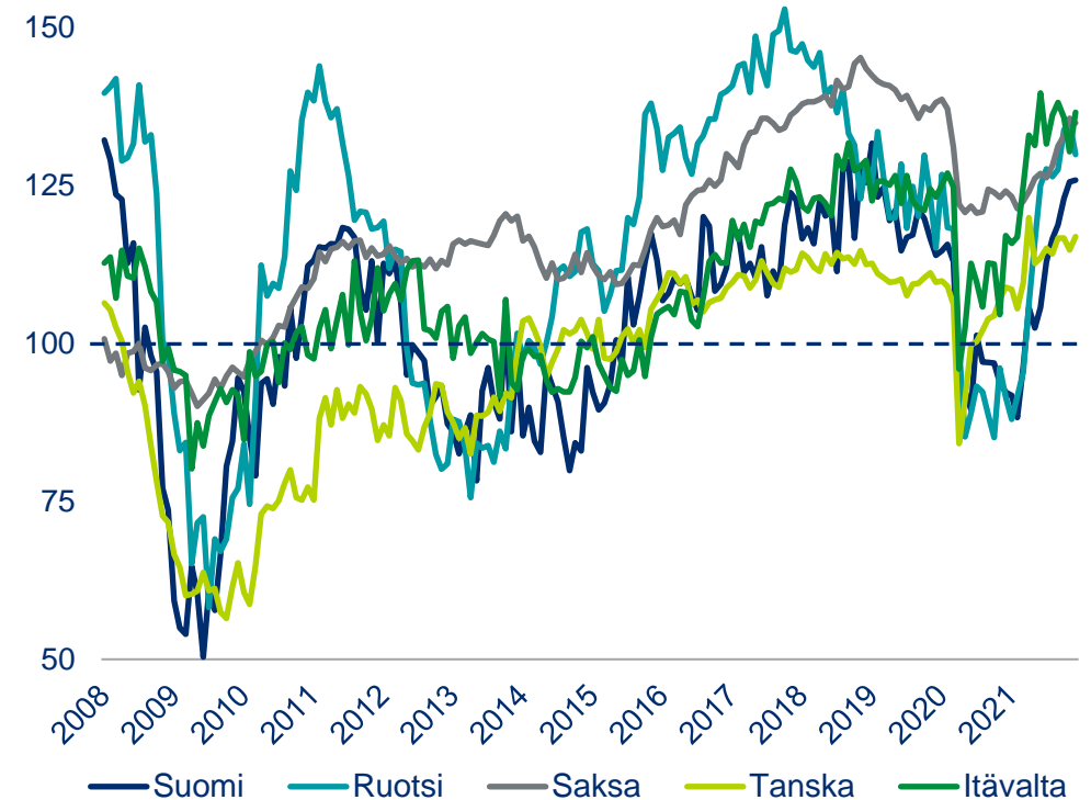
RAKENTAMISEN LUOTTAMUSINDIKAATTORI (2008 – 12/2021)
