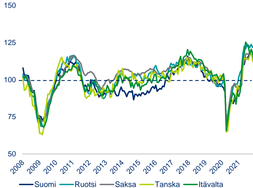
YLEISTALOUDELLINEN LUOTTAMUSINDIKAATTORI (2008 – 12/2021)
