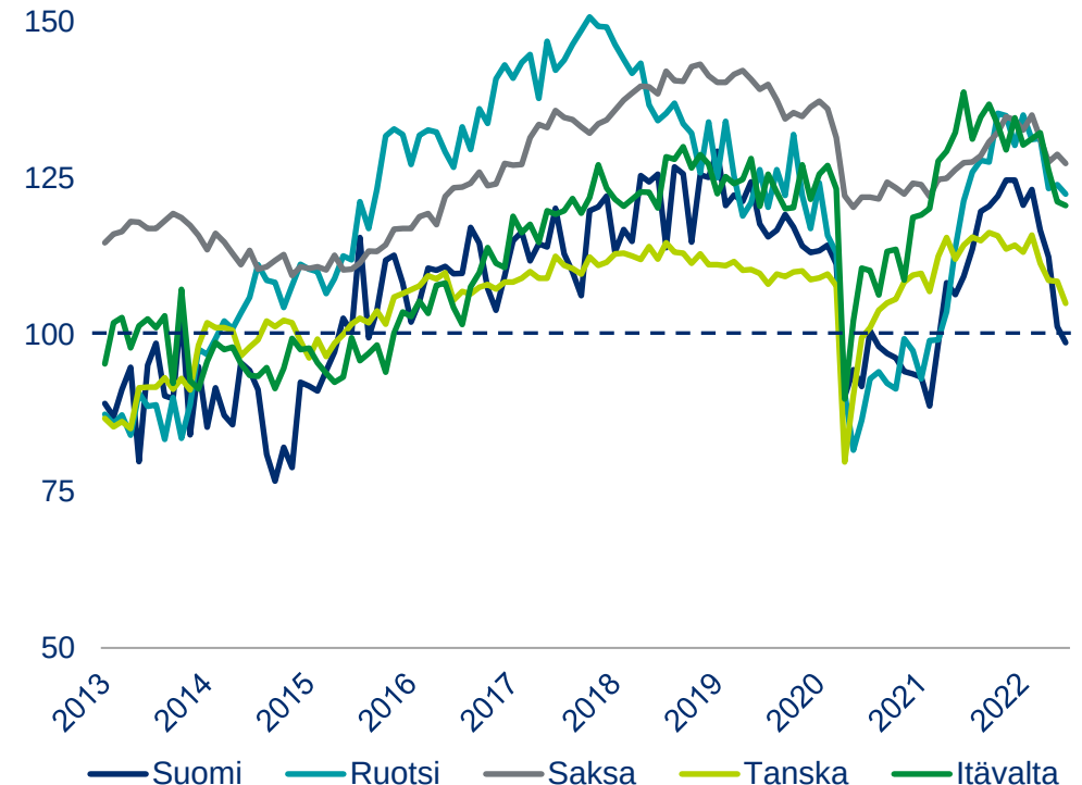
RAKENTAMISEN LUOTTAMUSINDIKAATTORI (2013 – 06/2022)
