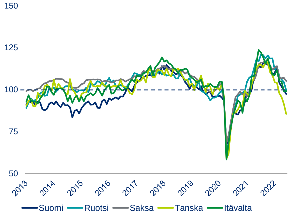
YLEISTALOUDELLINEN LUOTTAMUSINDIKAATTORI (2013 – 06/2022)
